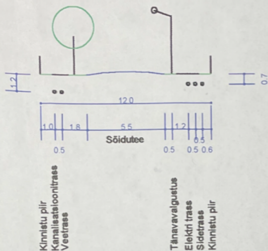
Tänavaristlõige 1-1
