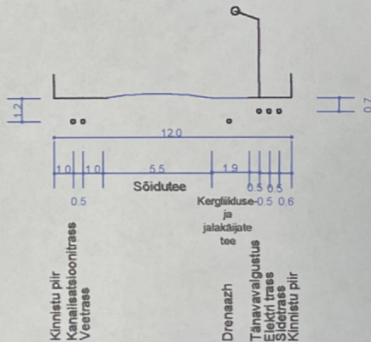
Tänavaristlõige 4-4
