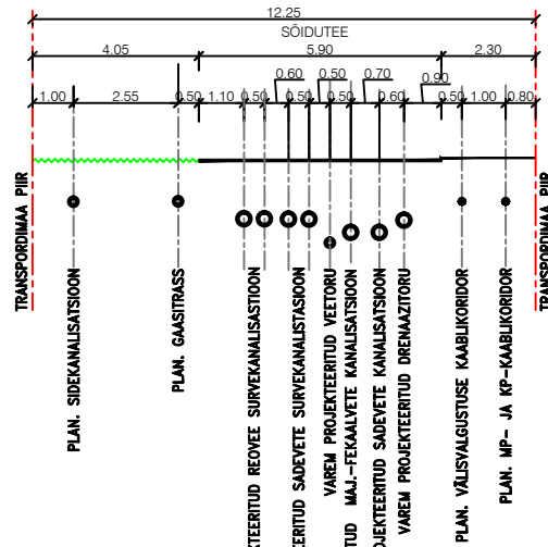
LÕIGE 1-1 M 1:100
