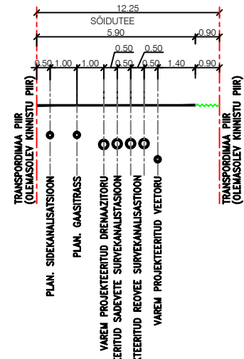
LÕIGE 2-2 M 1:100
