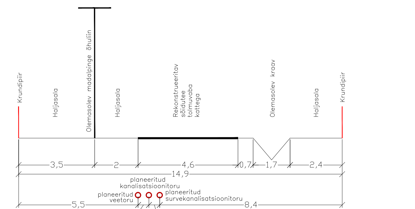
LÖIGE 2-2 TEE RISTLÖIGE M 1:100
