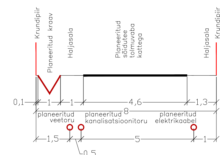
LÖIGE 2-2 TEE RISTLÖIGE M 1:100
