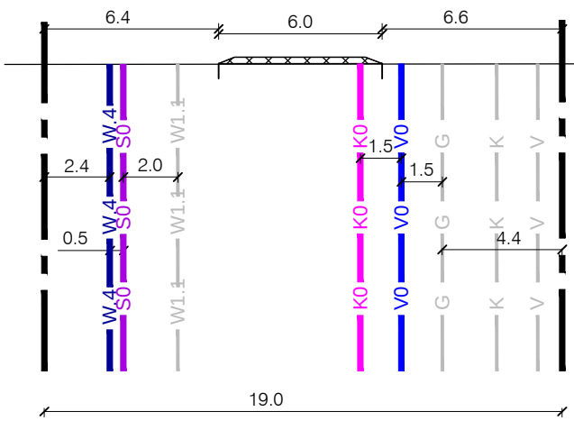
Lõige A-A
