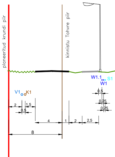
TEE RISTLÕIGE 3 - 3
