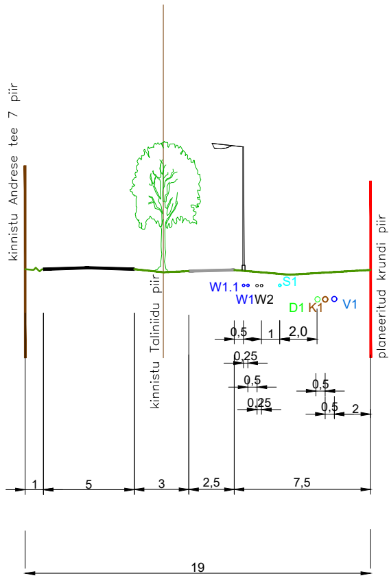
TEE RISTLÕIGE 3 - 3
