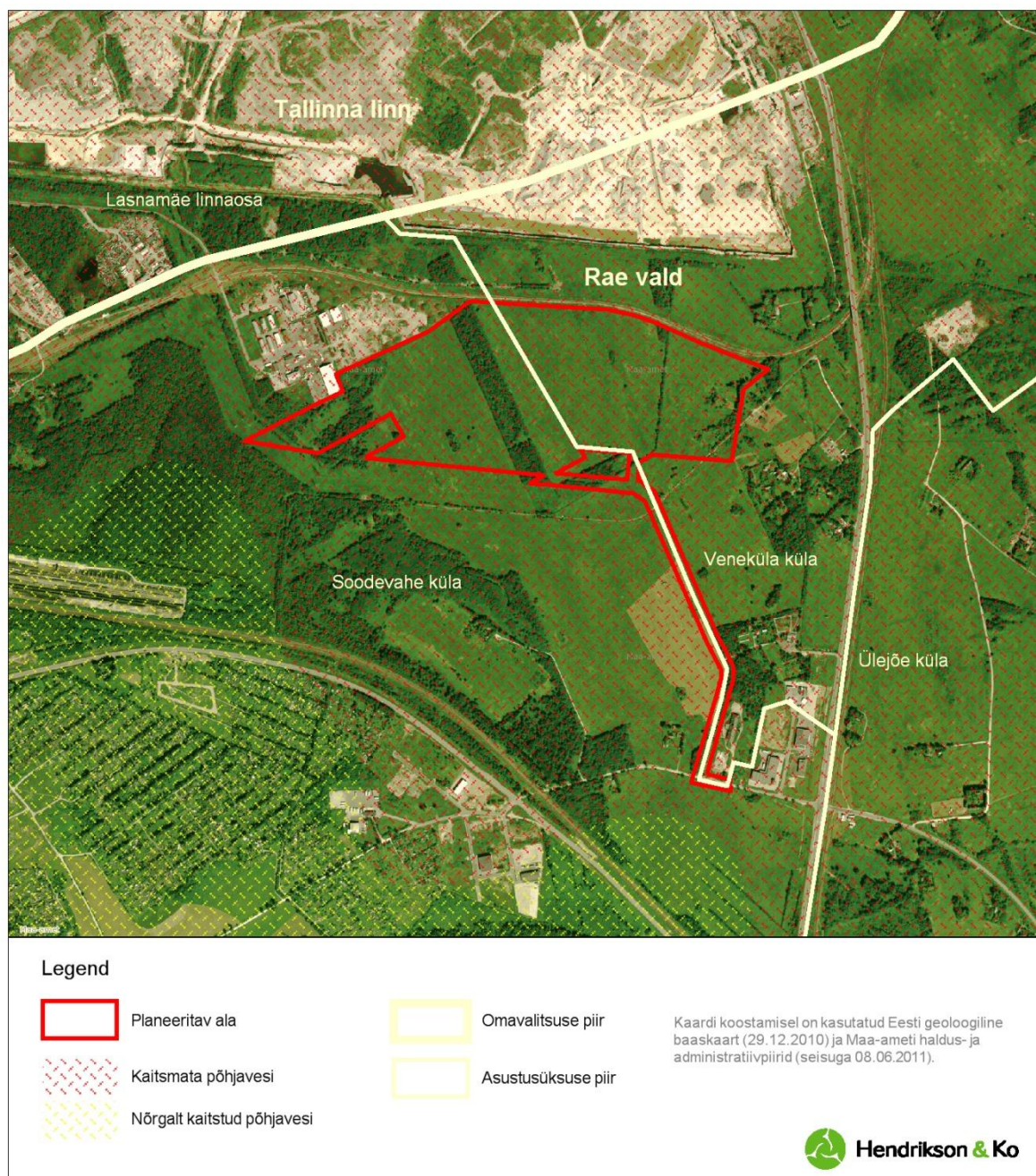
Joonis 4.2. Planeeringuala põhjavee kaitstus. Allikas: Maa-ameti geoloogia kaardirakendus.
