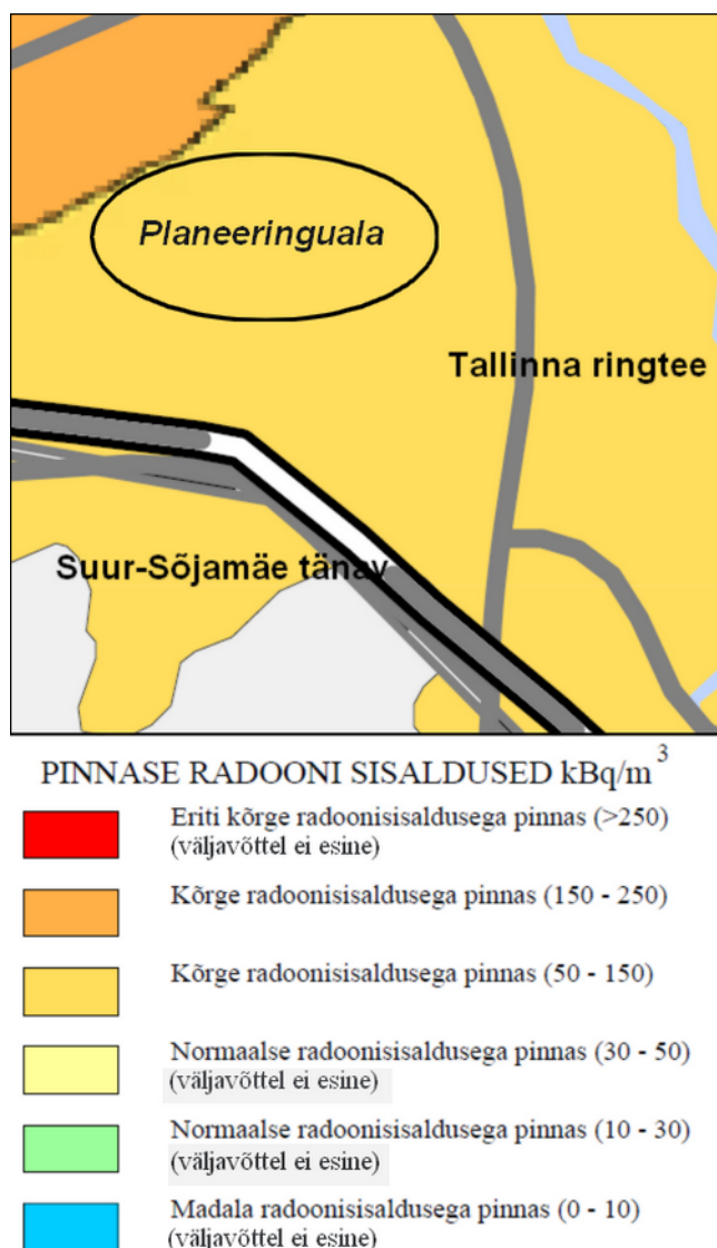
Joonis 4.5. Väljavõtte Harjumaa radoonikaardist planeeringuala ligikaudse paiknemisega. Kaardi koostaja: Eesti Geoloogiakeskus.
