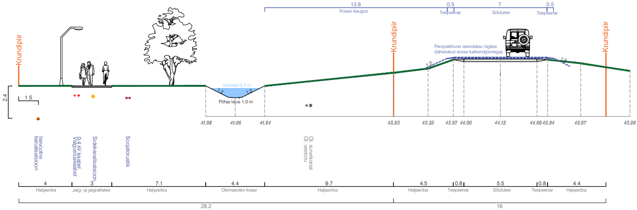
LÕIGE E-E' Kergliikluskoridor (Pos 35) koos perspektiivselt rekonstrueeritava riigiteega
