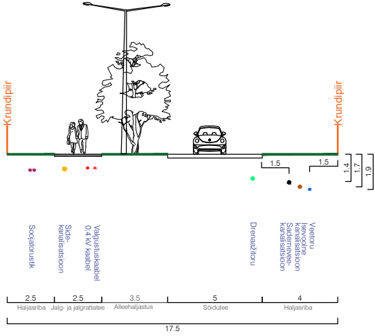
LÕIGE C-C' Pos 28
