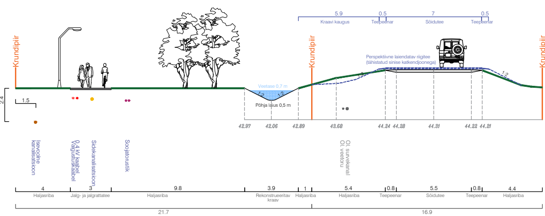
LÕIGE F-F' Kergliikluskoridor (Pos 35) koos perspektiivselt rekonstrueeritava riigiteega
