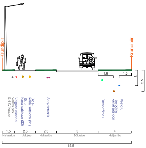
LÕIGE A-A' Tamme tee (Pos 30)
