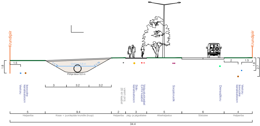
LÕIGE B-B' Pos 29
