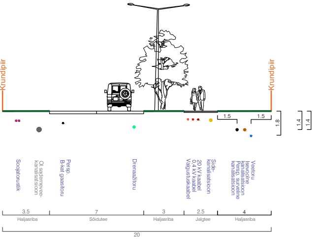
LÕIGE D-D' Kesk tee (Pos 27)
