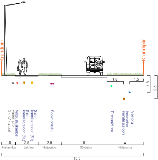
LÕIGE A-A' Tamme tee (Pos 30)
