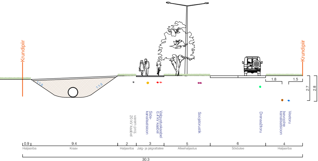
LÕIGE C-C' Pos 29
