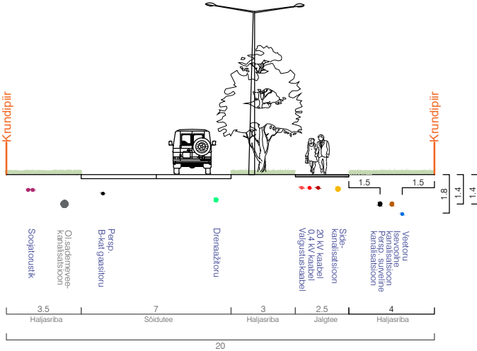
LÕIGE E-E' Kesk tee (Pos 27)
