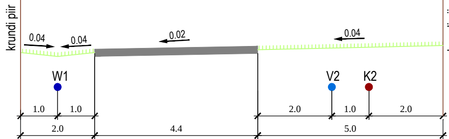
LÕIGE 1-1 M1:100
