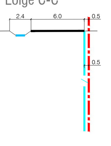
Lõige C-C
