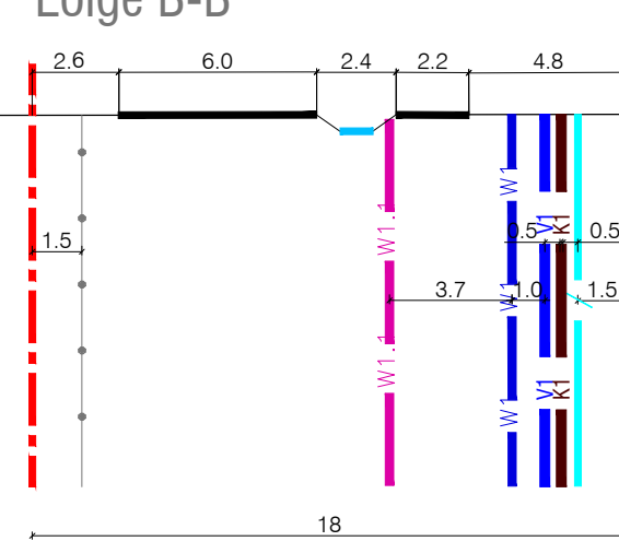
Lõige B-B
