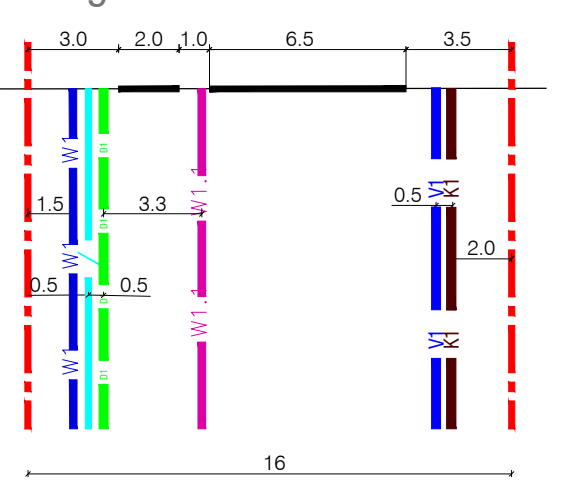
Lõige C-C
