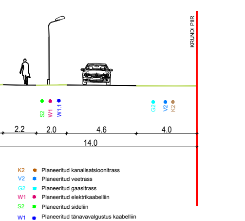
LÕIGE 4-4
