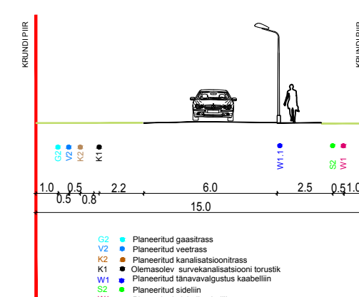
LÕIGE 3-3
