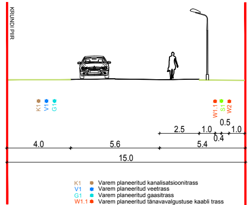
LÕIGE 2-2
