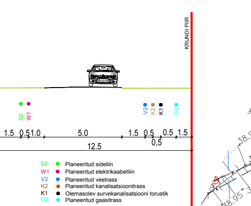
LÕIGE 4-4
