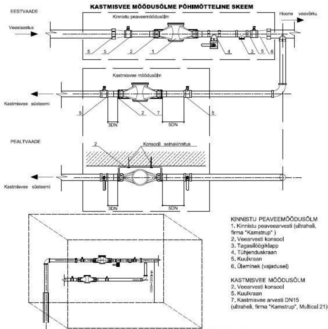
Kastmisveemöödusõlme põhimõtteline skeem
