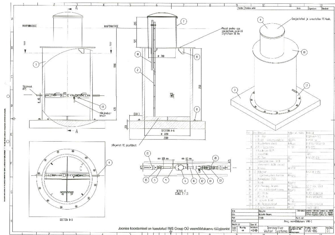
Veemõõdukaevu põhimõtteline skeem
