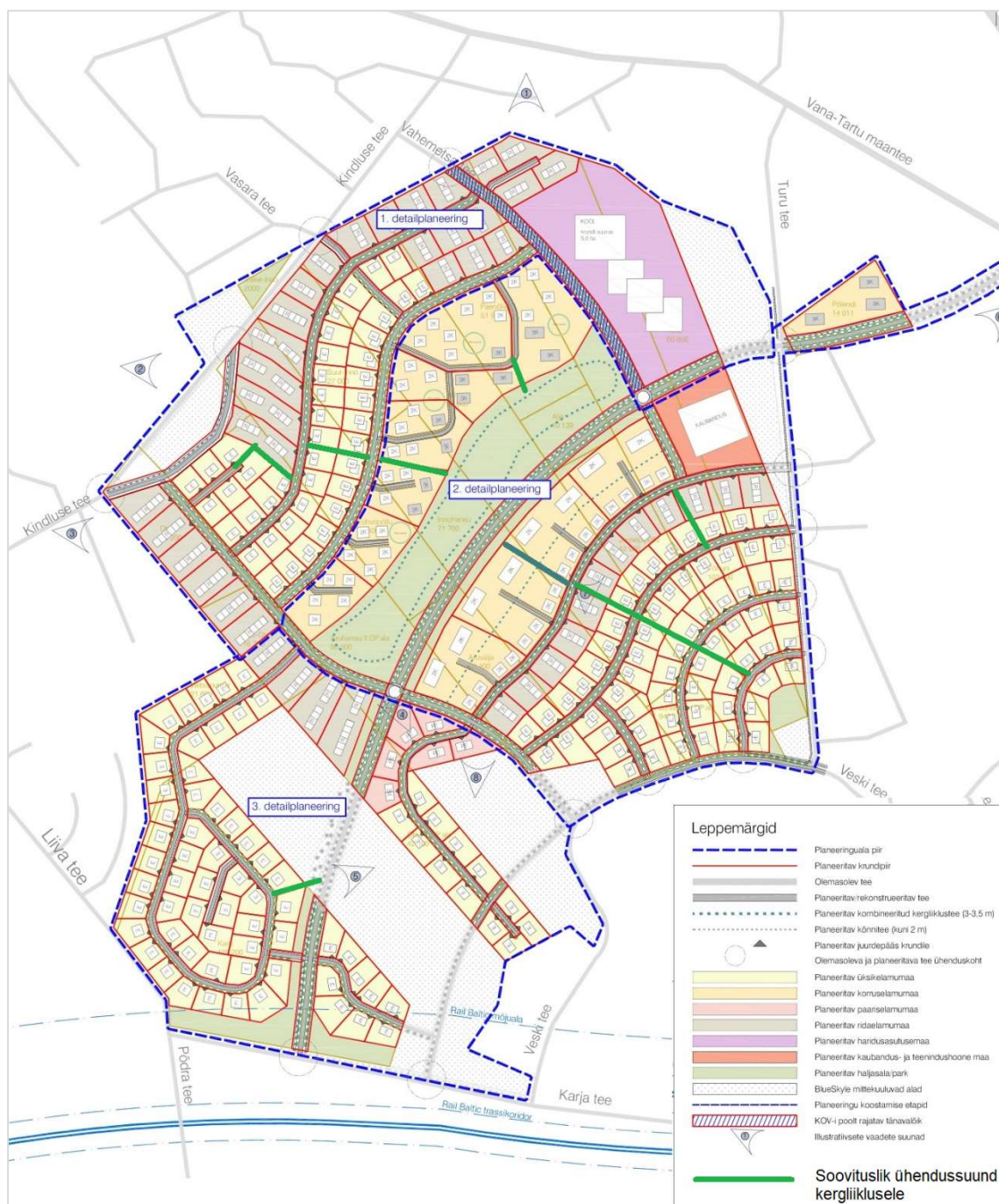
Joonis 3 Soovituslikud kergliikluse ühendussuunad planeeringualal
