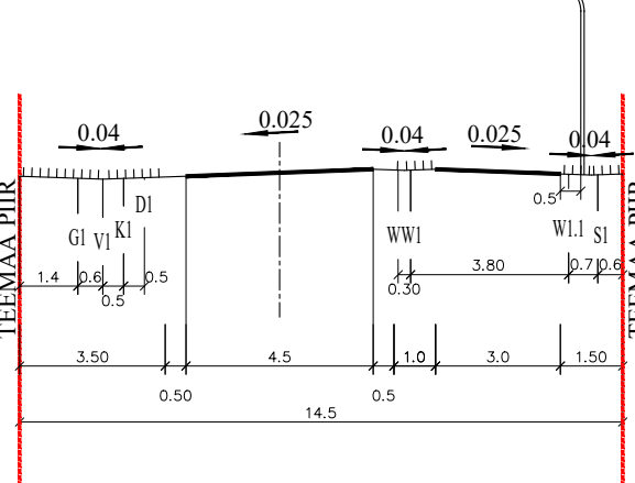
LÕIGE 2-2 M1:200
