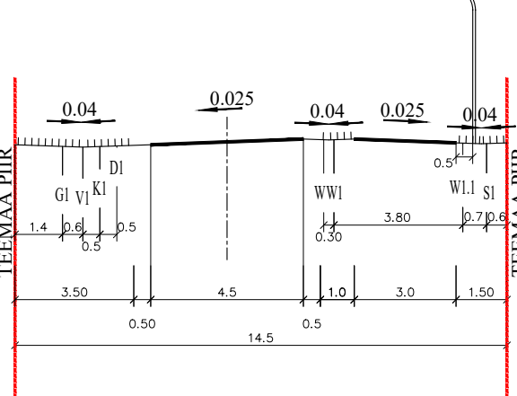
LÕIGE 4-4 M1:200
