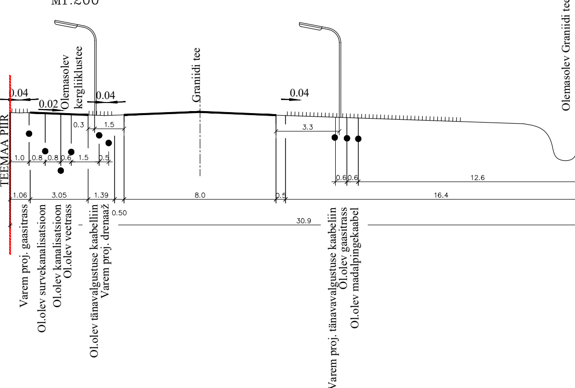
LÕIGE 7-7 M1:200
