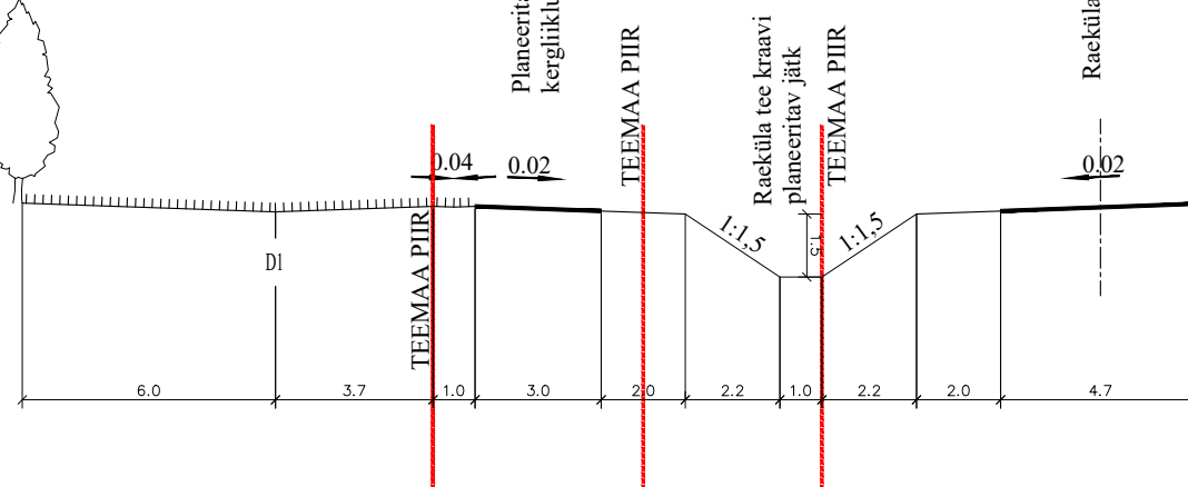
LÕIGE 7-7 M1:200
