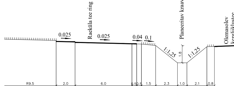
LÕIGE 8-8 M1:200
