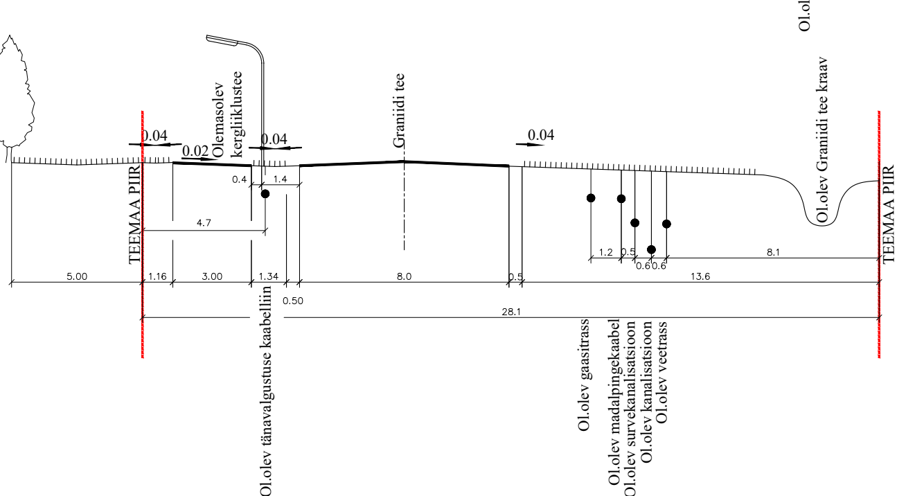
LÕIGE 6-6 M1:200
