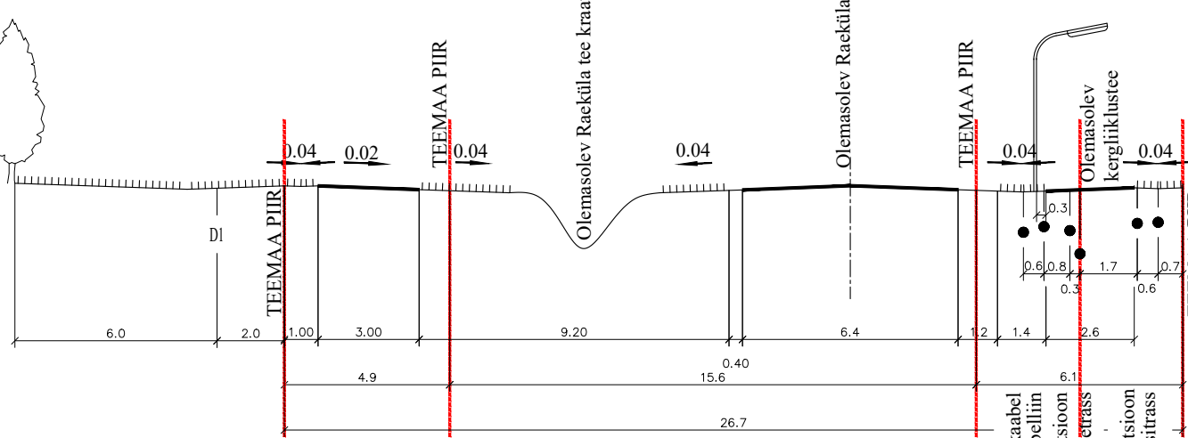
LÕIGE 4-4 M1:200
