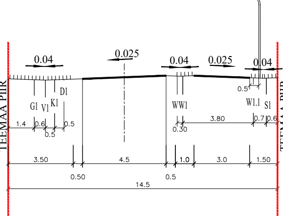
LÕIGE 1-1 M1:200
