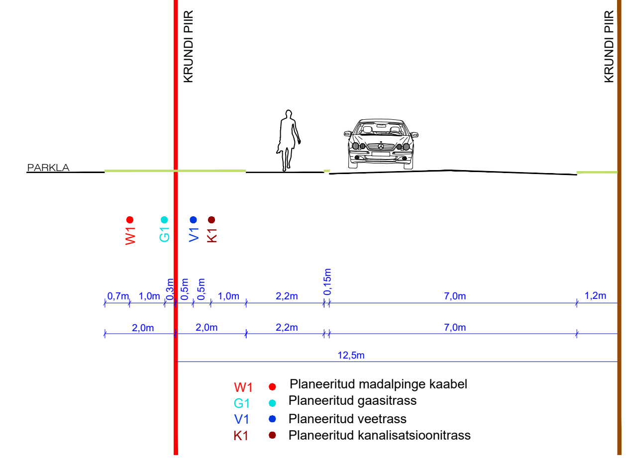
LÕIGE 2-2
