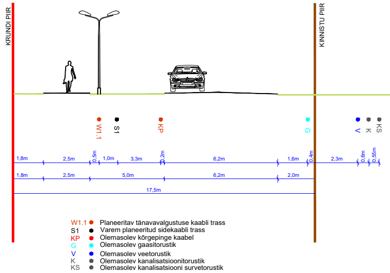
LÕIGE 3-3
