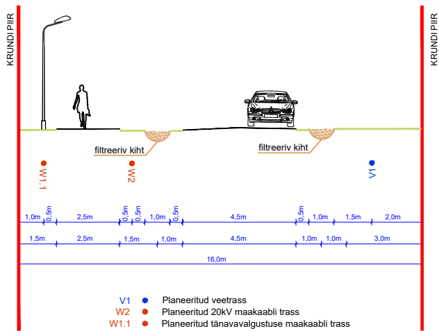
LÕIGE 5-5
