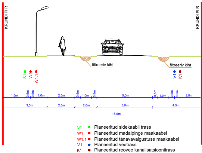
LÕIGE 3-3
