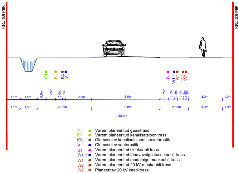
LÕIGE 4-4
