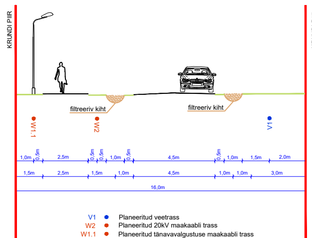
LÕIGE 4-4
