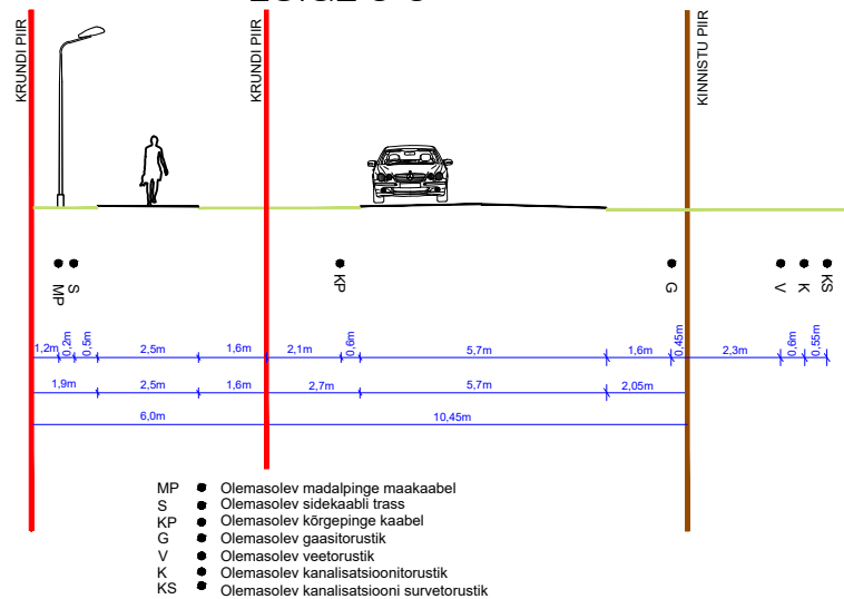
LÕIGE 3-3
