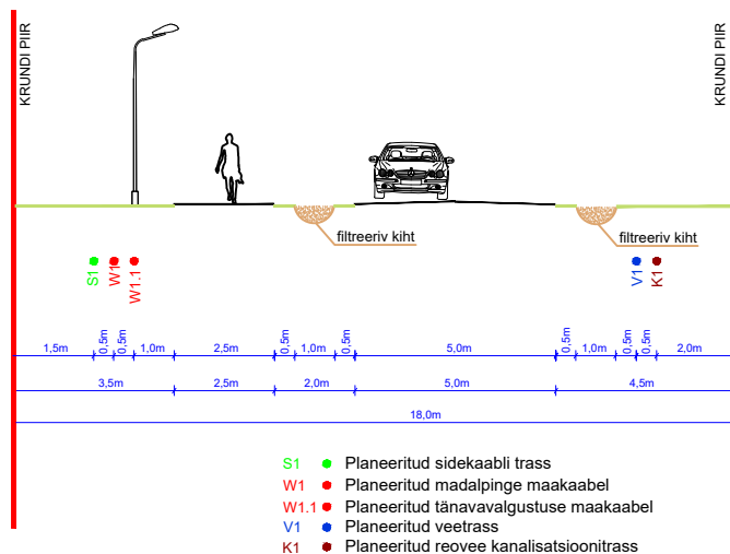
LÕIGE 3-3
