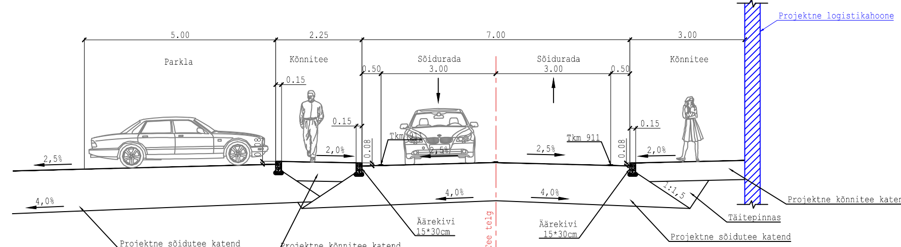
KINNISTU SISENE SÕIDUTEE KAHESUUNALISE LIIKLUSEGA, PARKIA JA LOGISTIKAHOONE VAHELISEL ALAL, KÖNNITEE KAHEL POOL TEED
