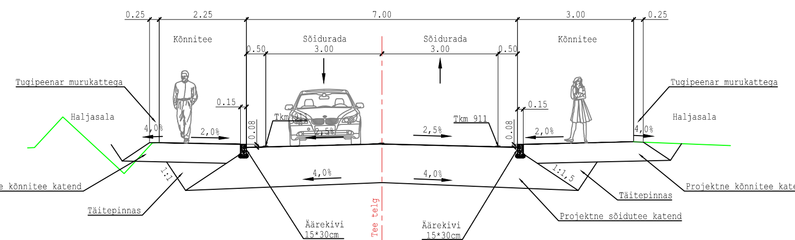
TÜÜPRISTPROFIIL B-B KINNISTU SISENE SÕIDUTEE KAHESUUNALISE LIIKLUSEGA, KÖNNITEE KAHEL POOL TEED
