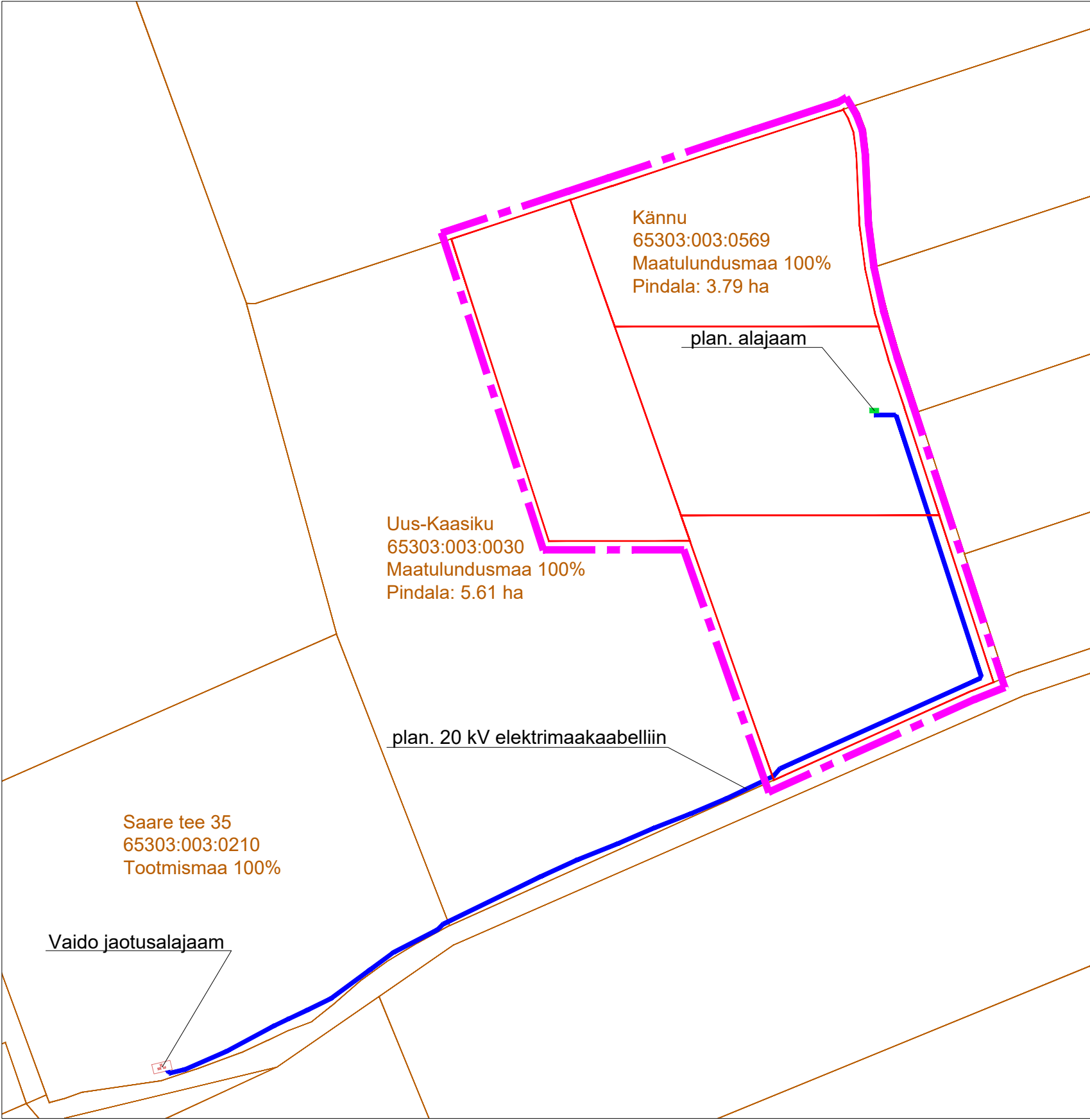
PLAN. 20 KV ELEKTRIMAAKAABELLIINI KULGEMISE SKHEM
