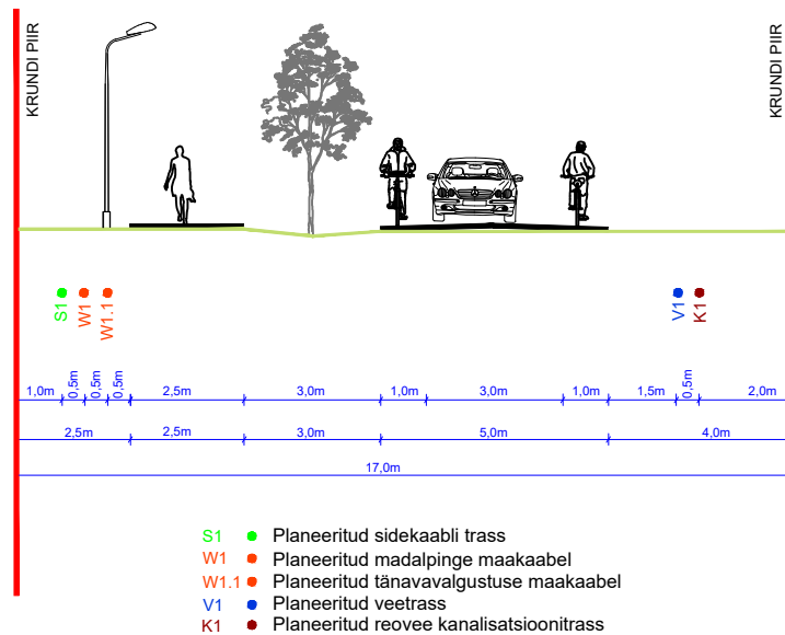
LÕIGE 1-1
