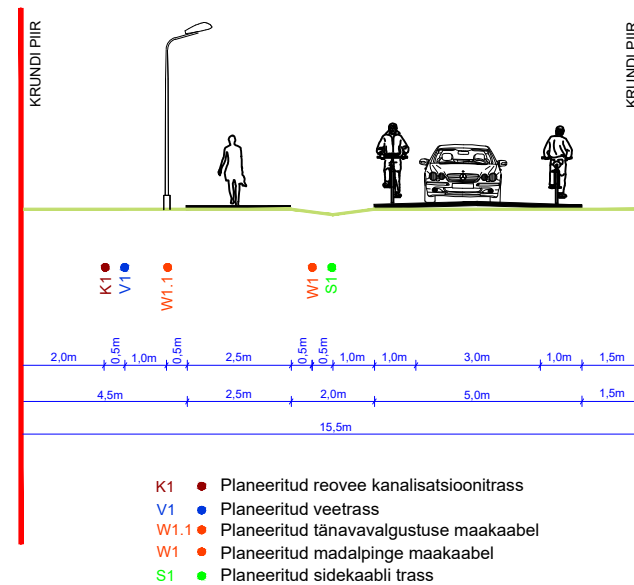
LÕIGE 2-2
