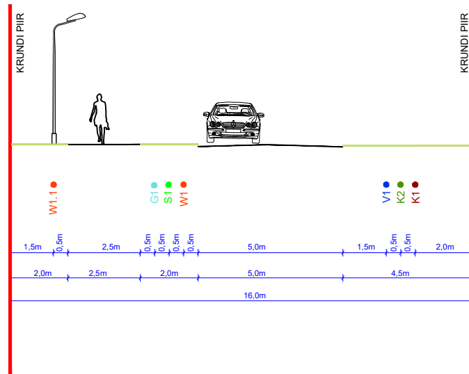
LÕIGE 3-3
