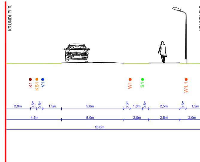
LÕIGE 5-5
