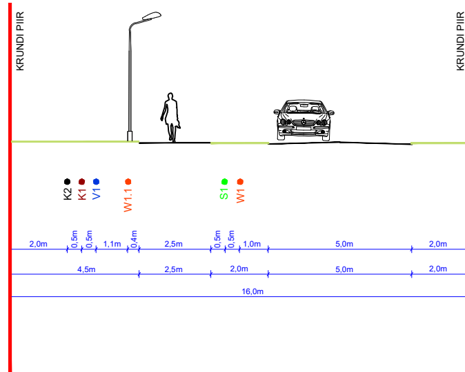
LÕIGE 1-1
