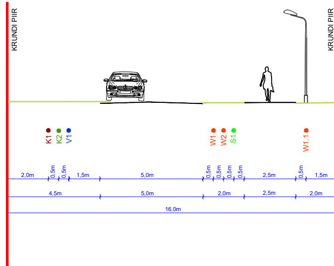
LÕIGE 2-2
