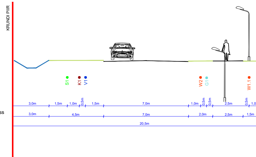
LÕIGE 4-4
