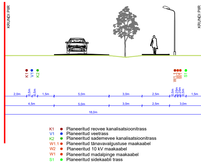
LÕIGE 2-2
