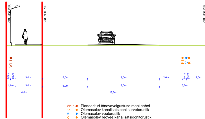
LÕIGE 3-3
