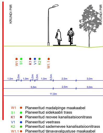
LÕIGE 1-1
