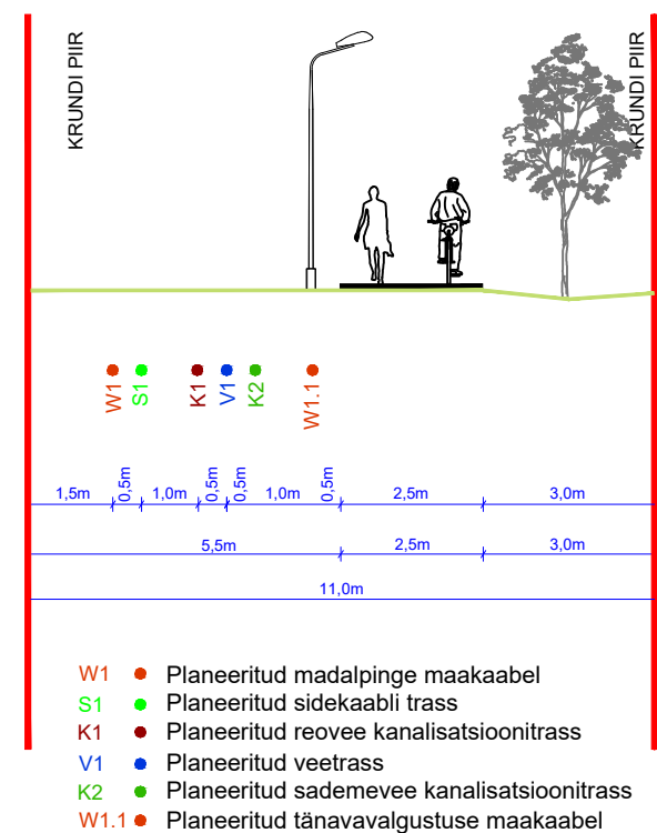
LÕIGE 1-1
