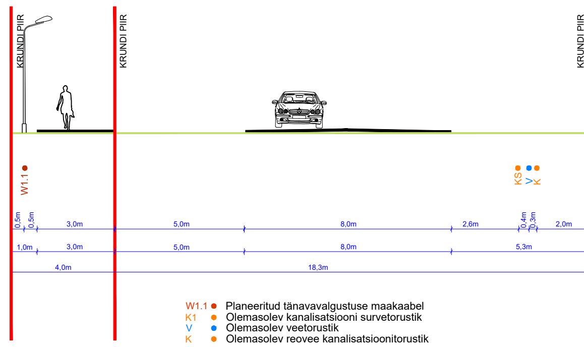
LÕIGE 3-3
