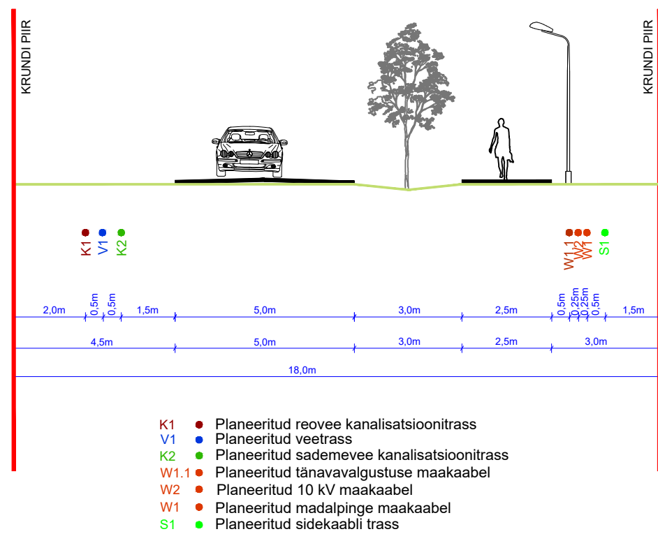
LÕIGE 2-2
