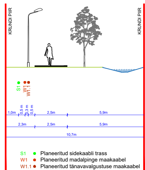
LÕIGE 2-2
