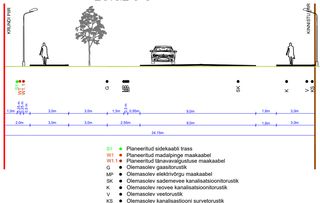
LÕIGE 3-3
