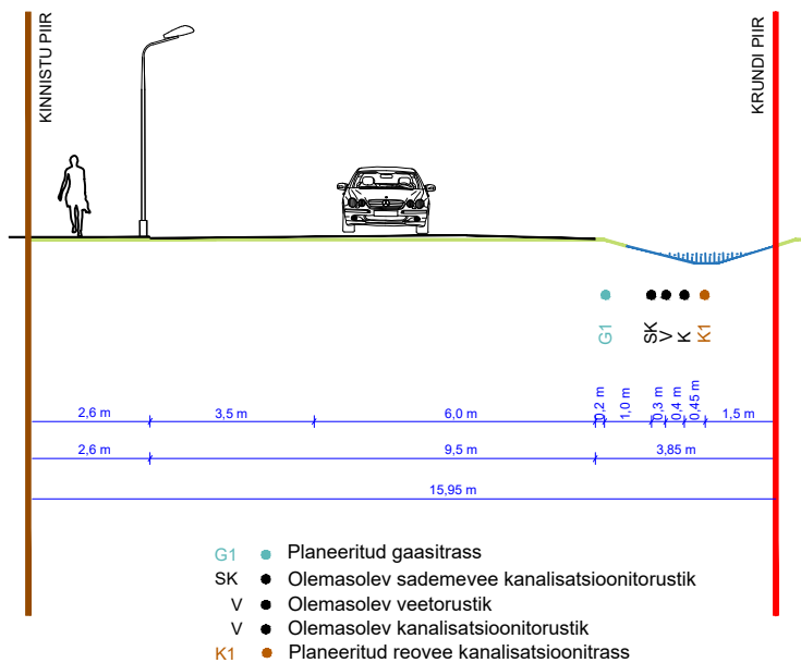
LÕIGE 1-1
